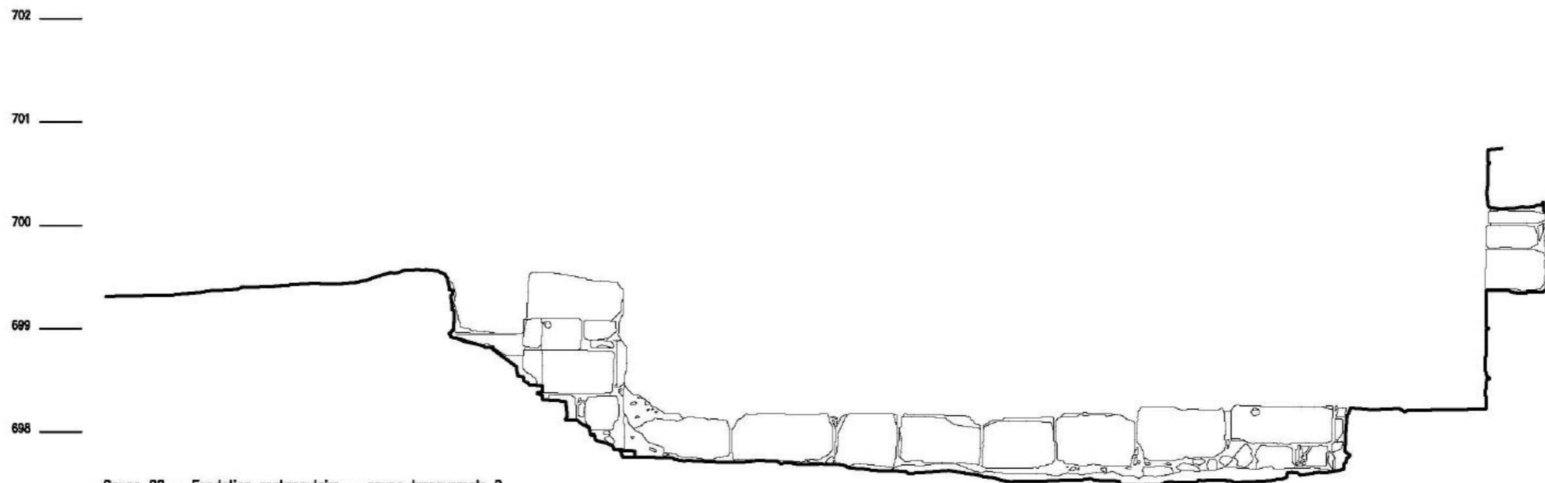
Coupe 22 - Fondation rectangulaire - coupe transversale 2 KHIRBET EDH DHARIH - Relevé Raphael Drizard - juillet/août 2001 - mise au net RD 2011
